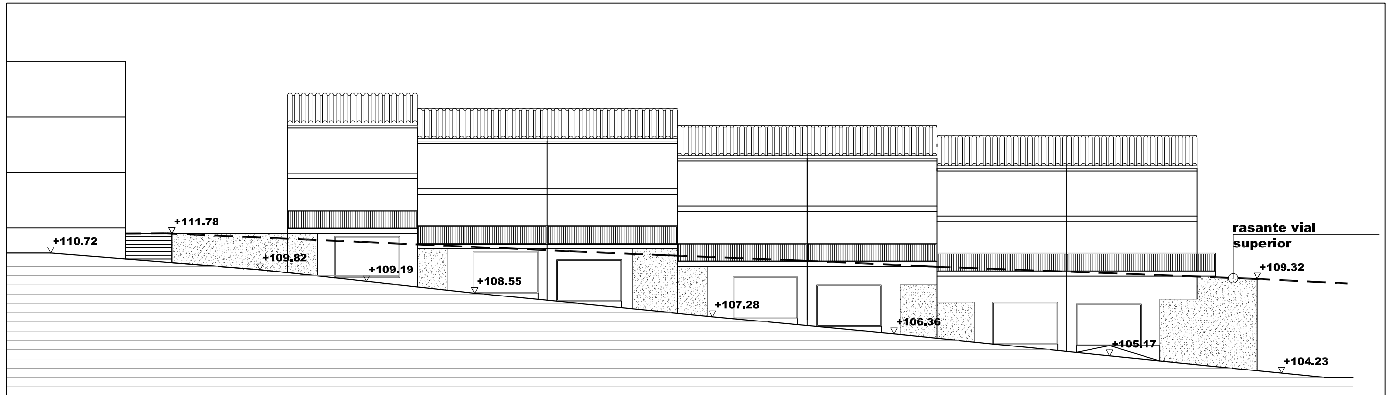
esquema de alzado noroeste
